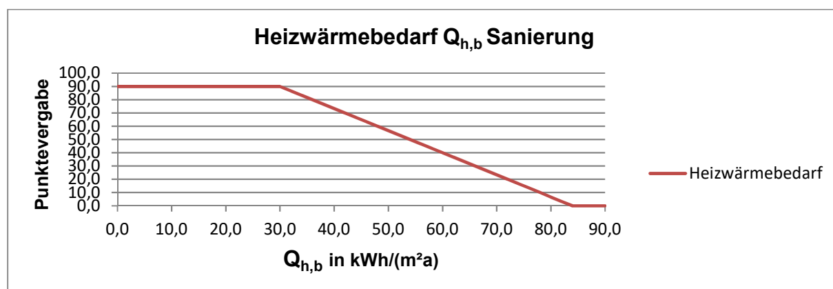
Grafik 14: Punktevergabe in Abhängigkeit vom Heizwärmebedarf
