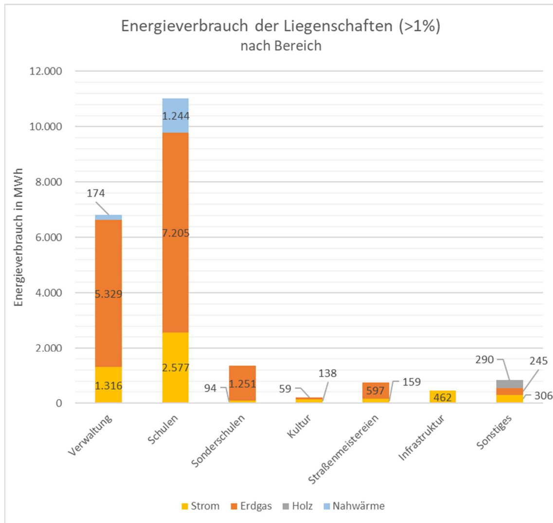
Abbildung 3: Energieverbrauch der Liegenschaften in 2021 nach Bereich (>1%) 7
