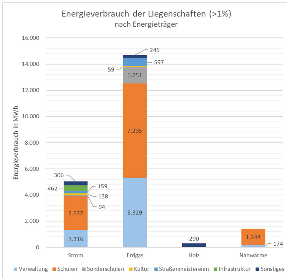
Abbildung 2: Energieverbrauch der Liegenschaften in 2021 nach Energieträger (>1%) 6
