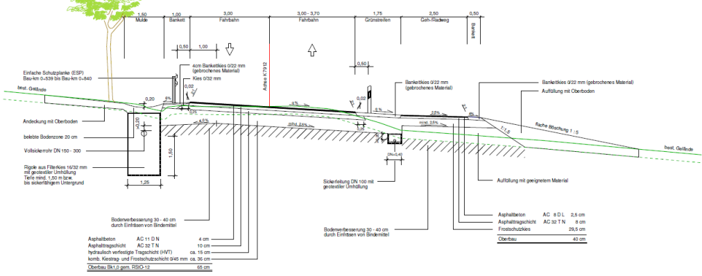
Kreisstraße K 7912 Bau-km 0+430 bis Bau-km 0+840
